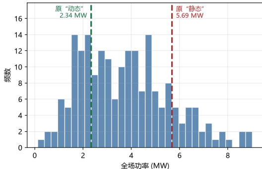
单一后端(FORIS)、零偏航、无策略 仅 reset 抽签 200 次的功率分布
